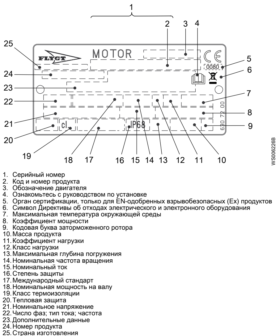
Рис. 6: Табличка для приводного блока начиная с 990101
