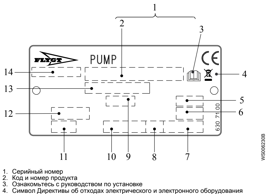
Рис. 6: Табличка для приводного блока начиная с 990101
