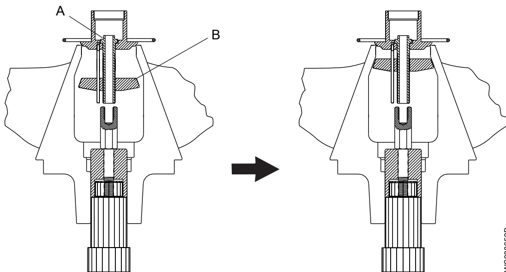
Рис. 36: Монтаж съемника
