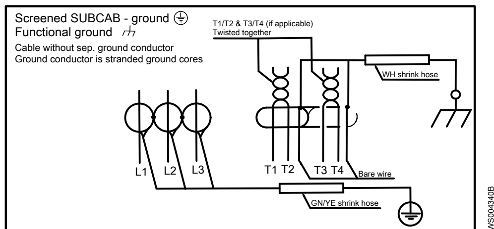
Рис. 22: Без отдельного провода заземления.
