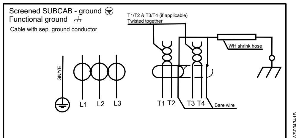
Рис. 23: С действующим заземлением
