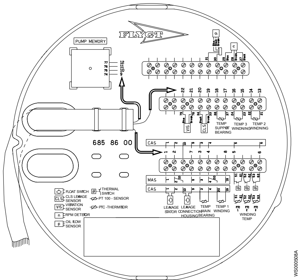
Рис. 17: Подключения устройства. Стрелки указывают номера проводов кабеля SUBCAB
